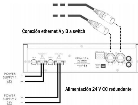
Vista posterior y ejemplo de conexión redundante de alimentación y red ethernet
